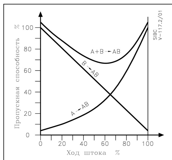
Рис. 4. Логарифмически / линейная характеристика регулирования (трехходовой клапан).
