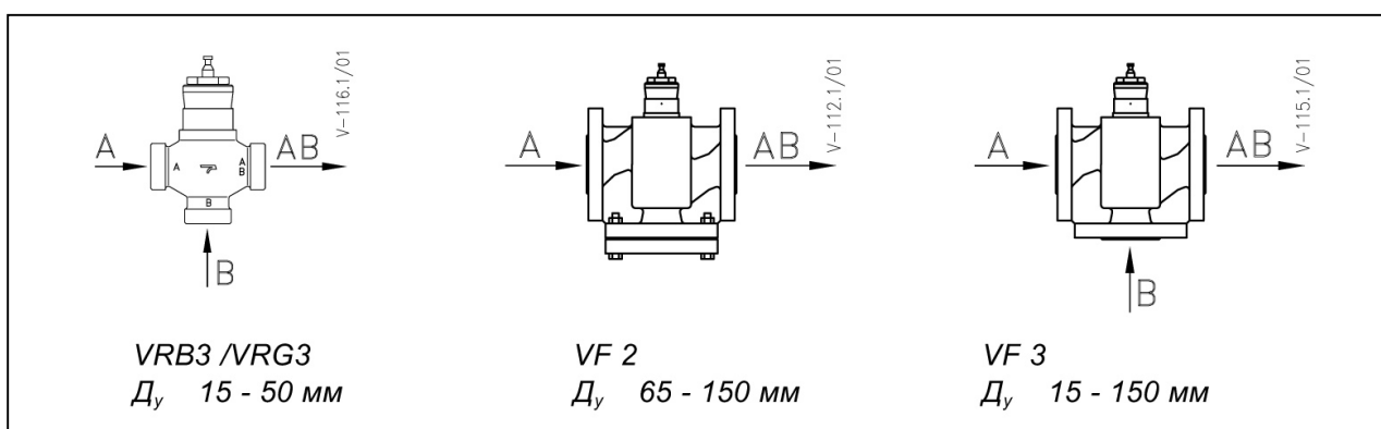
Рис. 5. Маркировка клапанов.
